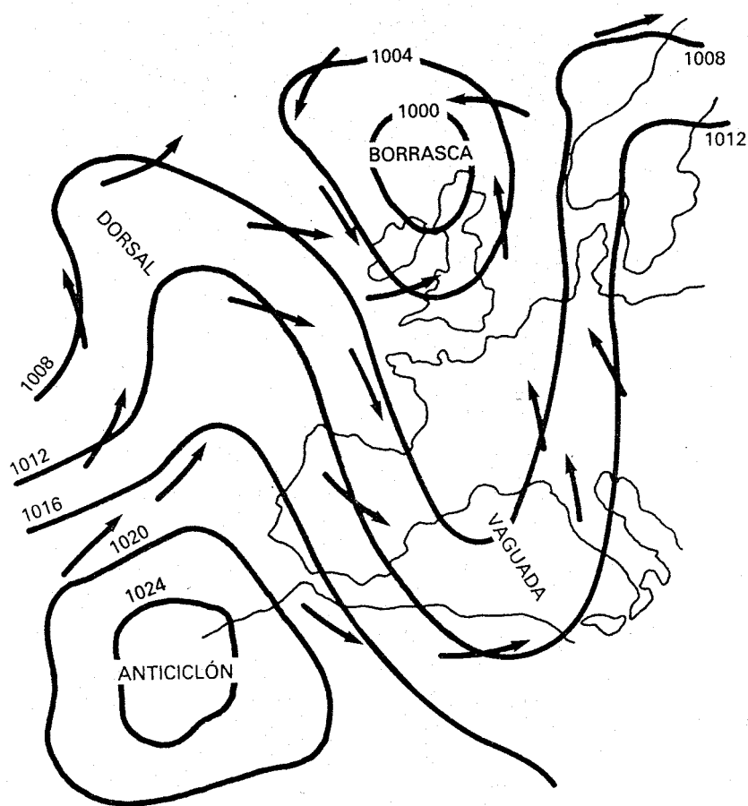
Fig. 4.1. Principales individuos isobáricos.
