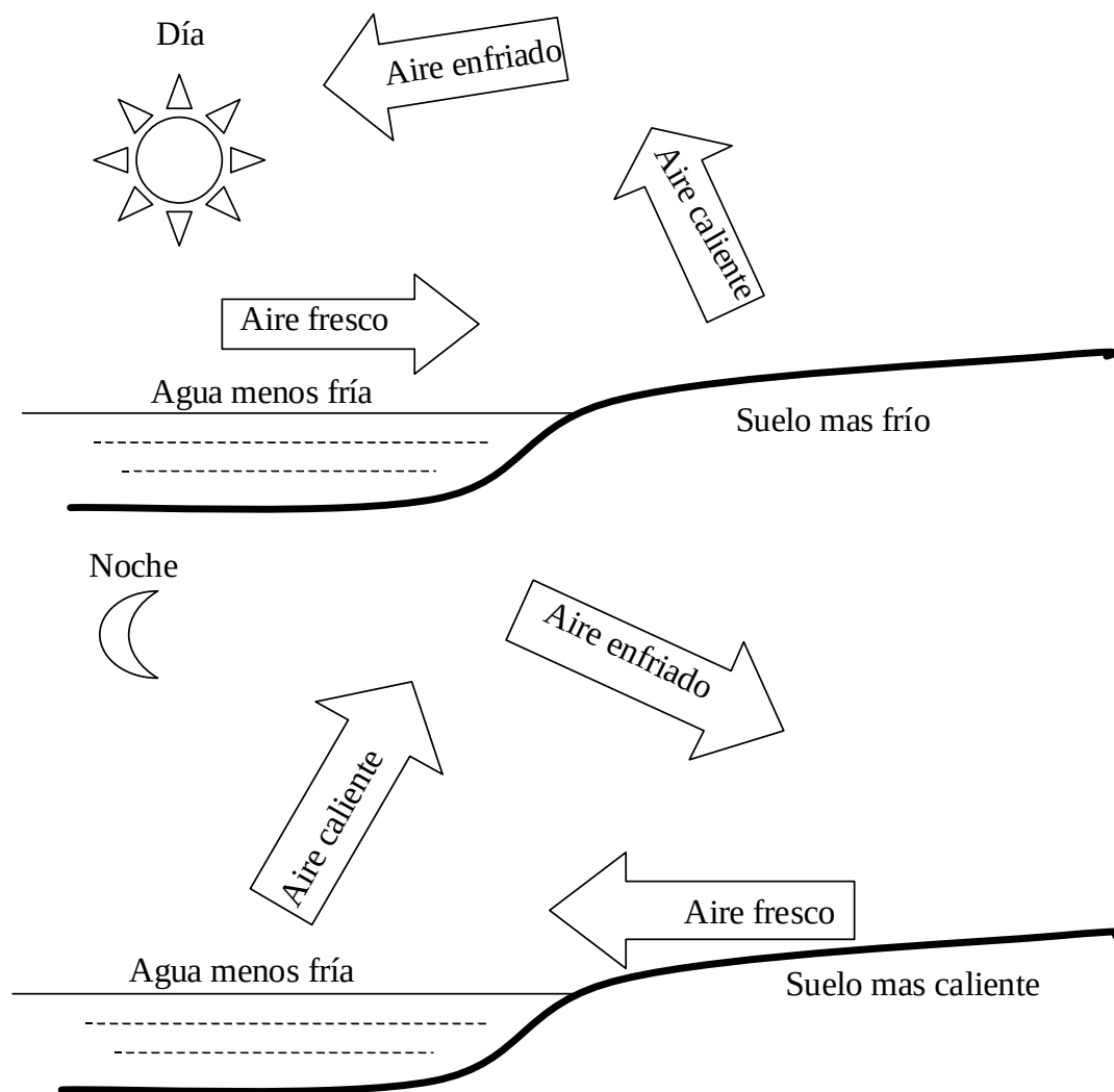
Fig. 5.7. Brisas de mar y de tierra.
