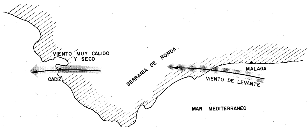
Fig. 6.3. Efecto Foëhn en la Serranía de Ronda (De Fuentes Yagüe, J.L, Mundi-Prensa, 1989).
