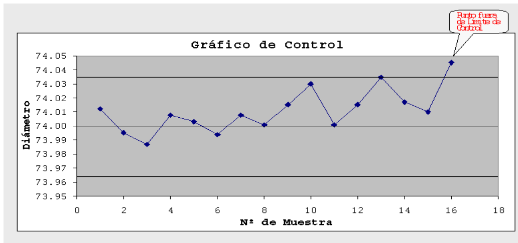
Figura 3. Diagrama de control. (González González & Jimeno Bernal, 2012)
