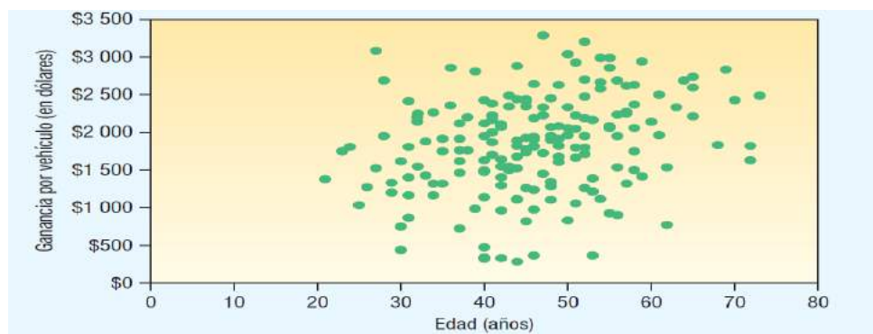
Figura 5. Diagrama de dispersión. (Lind, Marchal, & Wathen, 2015)
