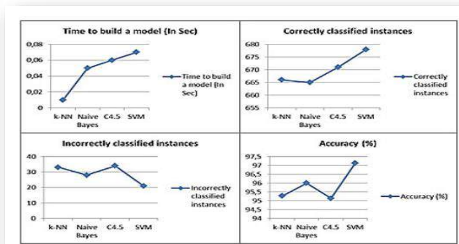
Figura 10. Gráfico comparativo de diferentes clasificadores. (Asri, Mousannif, Moatassime, & Noeld, 2016)
