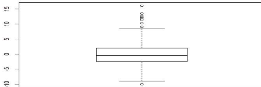
Figura 11. Diagrama de caja boxplot del caso autos. (Pizarro, Regresión lineal de autos, 2020)
