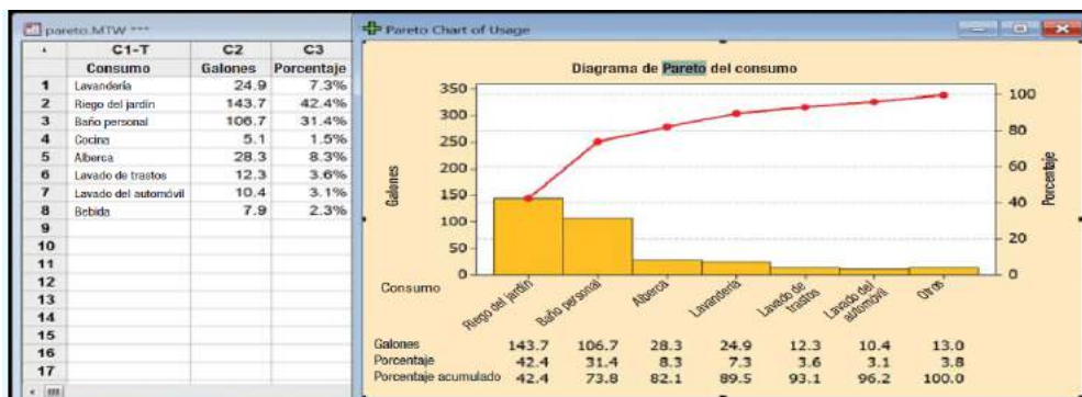
Figura 4. Diagrama de Pareto. (Lind, Marchal, & Wathen, 2015)
