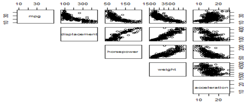
Figura 9. Correlaciones entre variables de los datos usando pairs() (Pizarro, Regresión lineal de autos, 2020).
