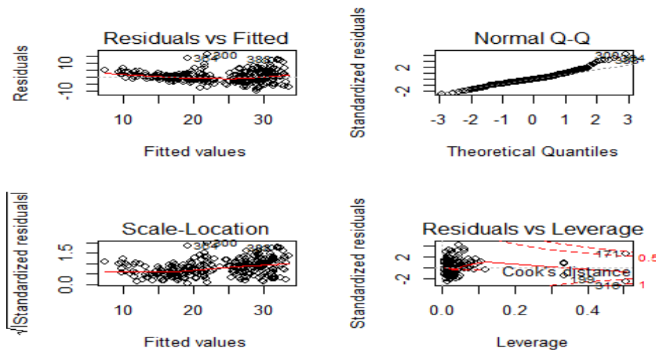
Figura 12. Varias gráficas del modelo de regresión. (Pizarro, Regresión lineal de autos, 2020)
