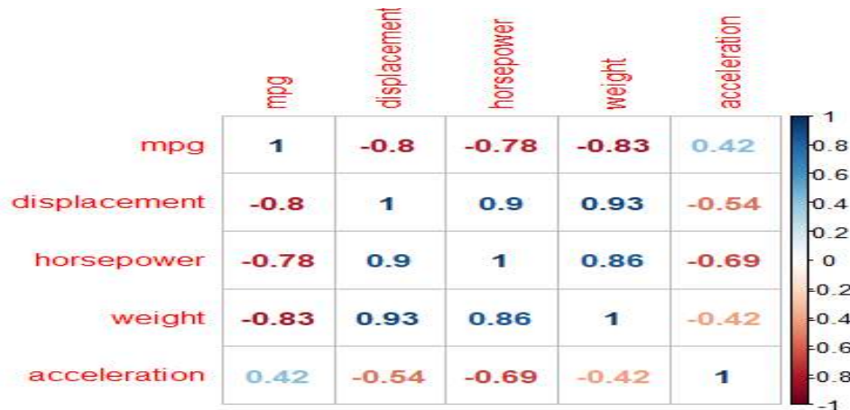
Figura 10. Correlaciones entre variables de los datos usando pairs() (Pizarro, Regresión lineal de autos, 2020).
